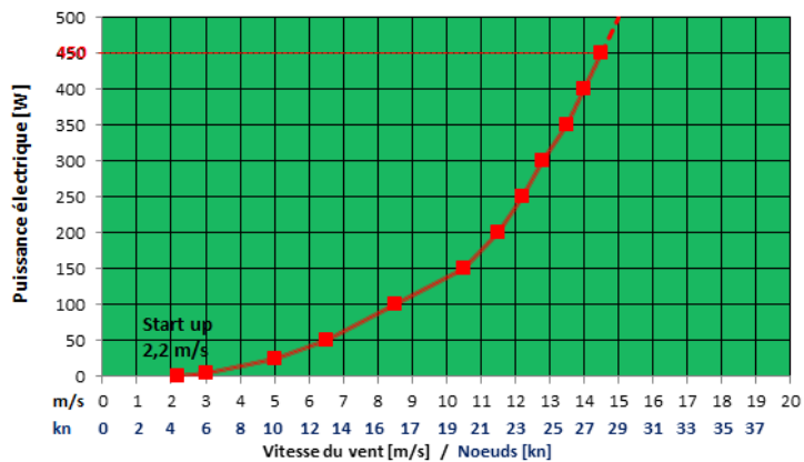
Courbe de performance* SILENTWIND 24V
