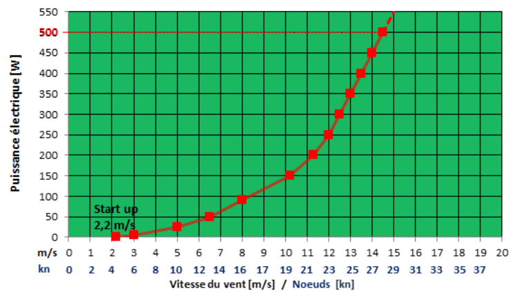
Courbe de performance* SILENTWIND 48V
