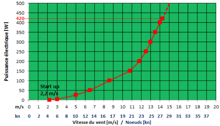
Courbe de performance* SILENTWIND 12V
